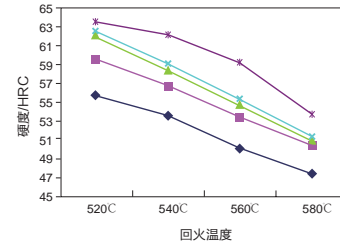
HSF210热处理曲线
